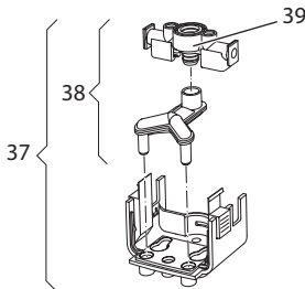
Abb. 23: Milcheinheit ausbauen
