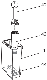
Abb. 24: Wasserfilter ein-/ ausschrauben
