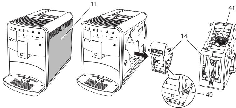
Abb. 22: Brühgruppe ausbauen
