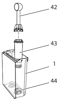
Fig. 24: Avvitare/svitare il filtro dell'acqua
