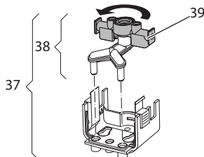
Abb. 21: Einlauf drehen
